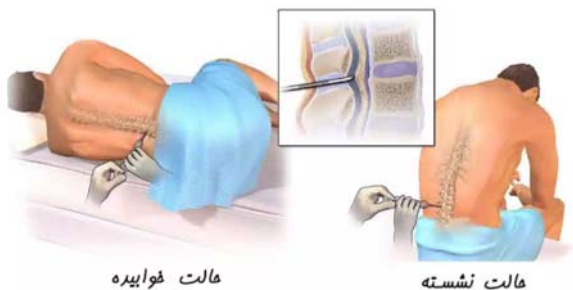
حالت های نمونه برداری از مایع مغزی نخاعی
